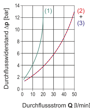
Δp-Q Kennlinien
