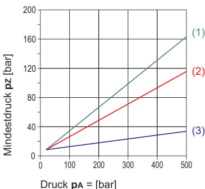
Mindestdruck p Z zum Entsperrn bei Druck p A (p B = 0 bar)
